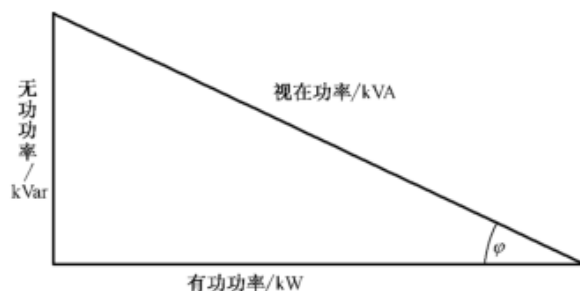
图1 功率三角形
