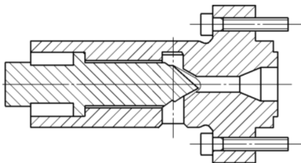
图3 II型试验喷嘴(未显示闭合装置)
