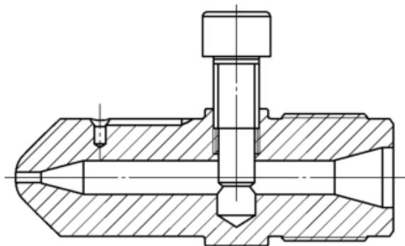
图2 I型试验喷嘴(未显示闭合装置)
